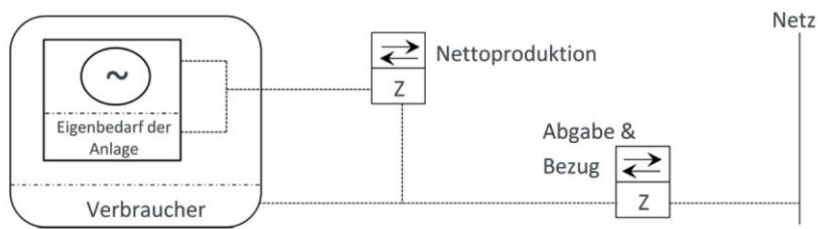
Abbildung 2 : Anordnung der Zähler bei Eigenverbrauch mit Anschlussleistung > 30 kVA
